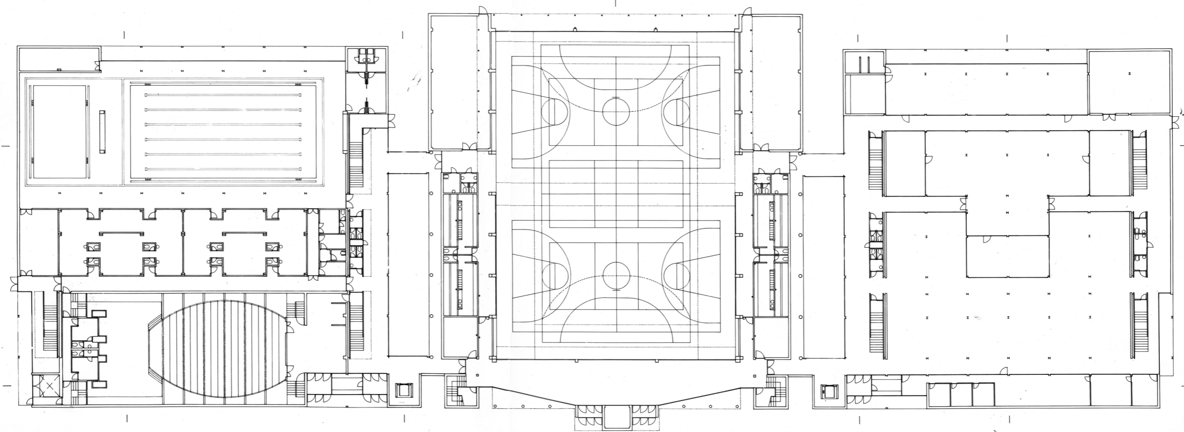
PLANTA BAJA GENERAL
